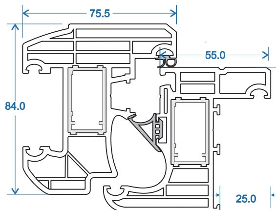
Sezione laterale
