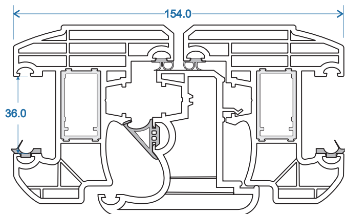
Sezione centrale
