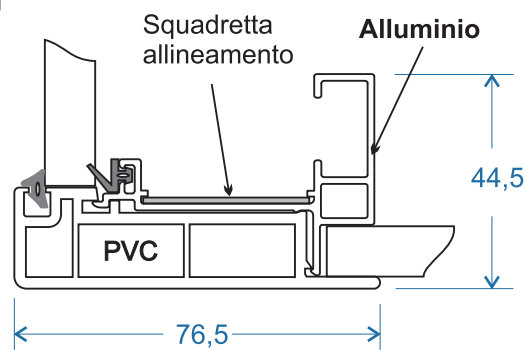
Profilo cassonetto
