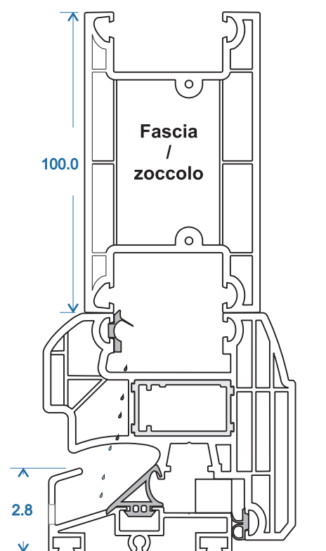
Soglia ribassata alluminio
