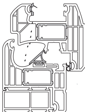
Riporto telaio
